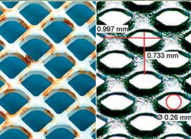
Im eigenen Prüflabor werden die Maschengrößen kontrolliert und das Streckgitter einem Salzsprühnebeltest unterzogen.
